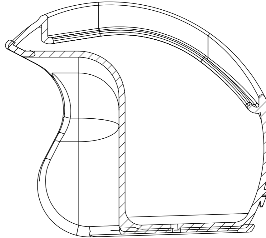
SECCIÓN A-A ESCALA 1 : 1
